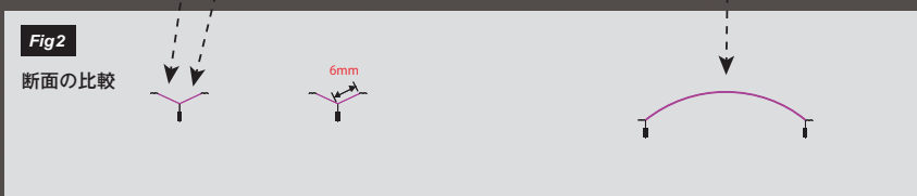
Fig2 はそれぞれのダイアフラムの断面を示しています。 CODA AUDIOのリングダイアフラムの幅は、一般的なダイアフラムに比べると狭く、この例では6mmとなります。
