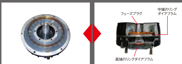
Fig1 同軸ドライバーの内部をイメージ
