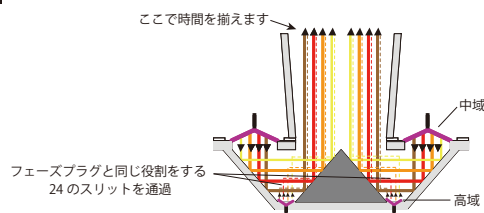
Fig1 同軸ドライバーの内部をイメージ
