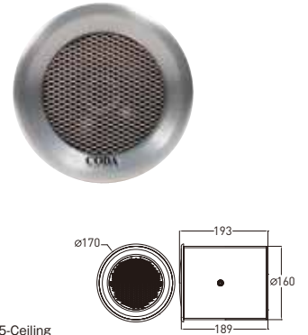
画像と寸法図はD5-Ceiling
