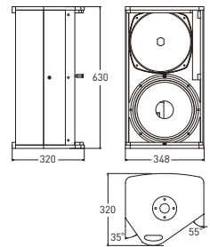
画像と寸法図は G712-96-R
