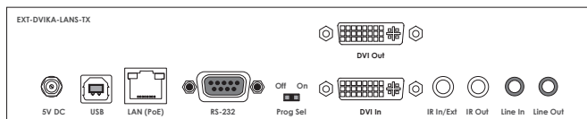
EXT-DVIKA-LANS-TX (送信機)
