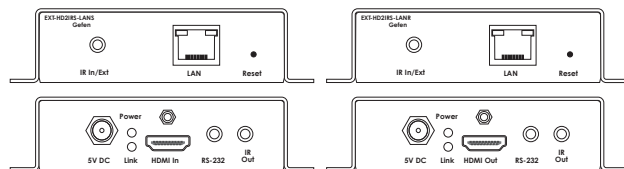
EXT-HD2IRS-LAN-TX (送信機) EXT-HD2IRS-LAN-RX (受信機)
