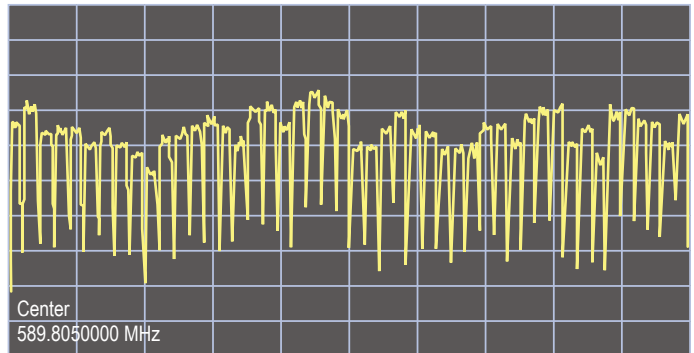
実際のスペクトラムスキャン結果。従来16チャンネルの運用であった周波数帯域で47チャンネルを運用できていることがわかります。(米国の周波数運用例)
