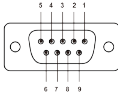
RS-232 Controller
