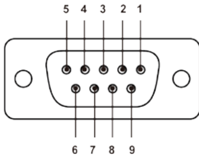
RS-232 Controller
