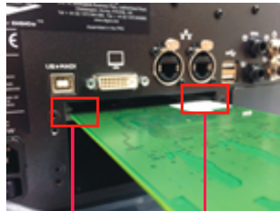
ガイドレールに合わせてカードを差し込む
