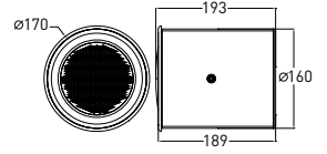
画像と寸法図はD5-Ceiling
