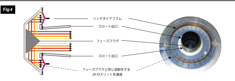
Fig4 実際のドライバーに当てはめます。画像は、ドライバーユニットからマグネットを外しています。
