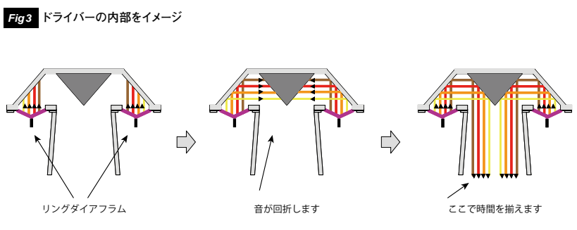
Fig3 リングダイアフラムの振動(音)がドライバー内部で回折して物理的に時間を揃えているため、優れた位相特性を備えています。このため、合理的な物理配置で音響デザインをすることが可能になります。
