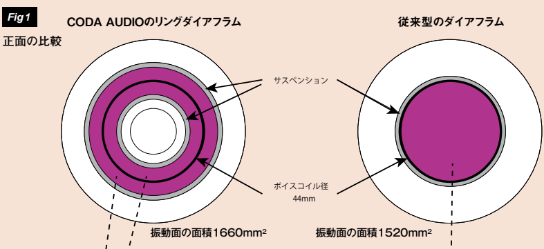
Fig1 に示すように、CODA AUDIOのリングダイアフラムは、内側と外側にサスペンションを備えています。 同じボイスコイル径で比較した場合、ピンクで示した振動面の面積はリングダイアフラムのほうが広くなります。
