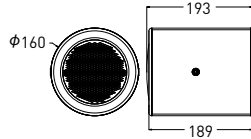
画像と寸法図はD5-Tube
