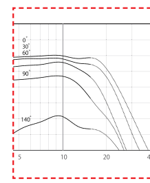
▲MMC4018VLの周波数特性
