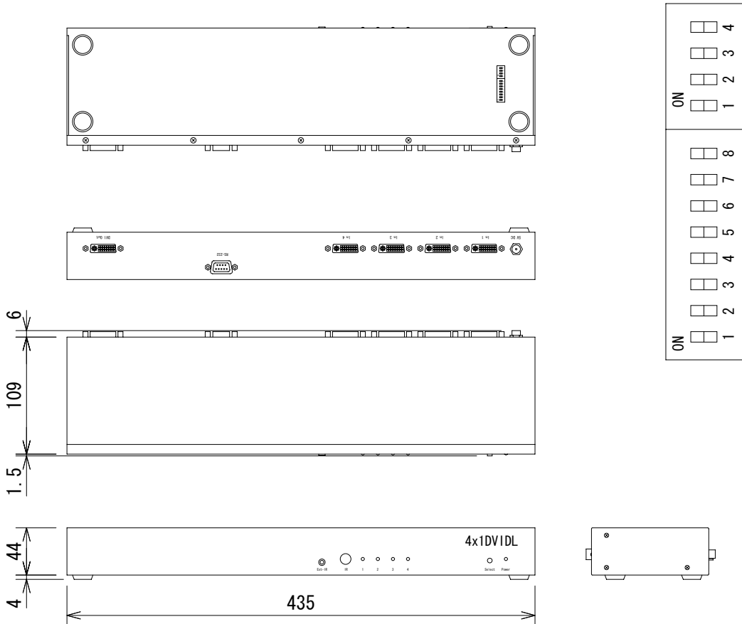
DIPスイッチ拡大図
