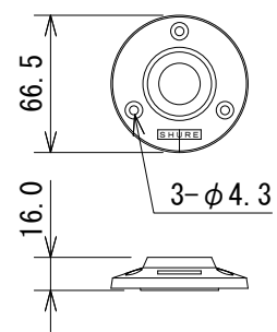
マウント用フランジ
