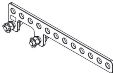
(図 15 EXBAR VR/FR-VR のエクステンションバー)
