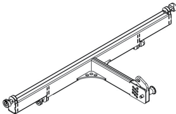
(図 16 DOW-VR 12/ViRAY を AIRLINE LA12 に連結する ダウンフィルフレーム)
