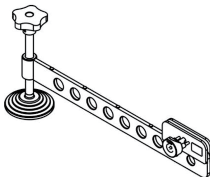
(図 18 TILT-VR/ViRAY と SCV-F のグラウンドスタック用傾斜金具)
