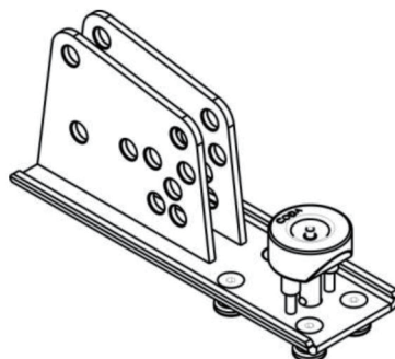
(図 17 VGA/ViRAY のグラウンドスタック用アダプター)
