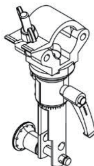
( 図 19 : VARIO CLAMP / AiRAY, ViRAY, N-RAY, TiRAY, APS, N-APS フレーム / エクステンションバー用仮設トラスクランプ )
