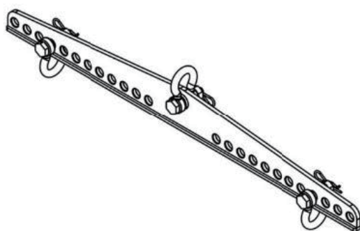
(図 15 : BAR-APS / APS 用水平アレイクラスターフレーム)
