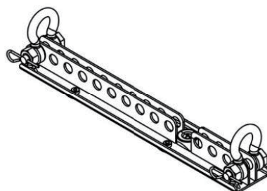
(図 13 : FRH-APS / APS の水平フライング用フレーム)
