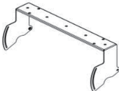
( 図 20 : AV-APS / APS 用天吊り U ブラケット )
