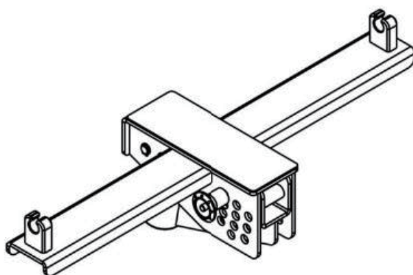
(図 16 : CU-APS / APS のグラウンドスタック用ディスタンスポールアダプター)
