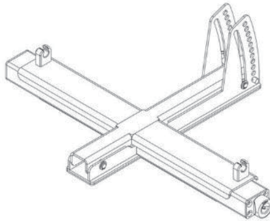
( 図 17 : GA-APS / APS、APS-SUB 用グラウンドスタックアダプター )
