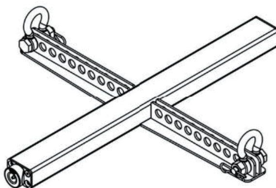
(図 12 : FRV-APS / APS、APS-SUB の垂直フライング用フレーム)
