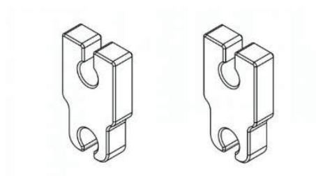
( 図 21 : FRV-DA-APS / APS/APS-SUB の垂直アレイ用プルバックアダプタ )
