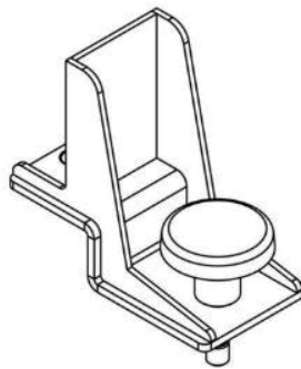
( 図 18 : GAH-APS / グラウンドスタッキングした APS-SUB 上に APS の水平アレイを載せるときに使用するアダプター )
