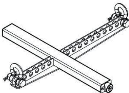
(図 12 : FRV-N-APS / N-APS 用垂直アレイフレーム)
