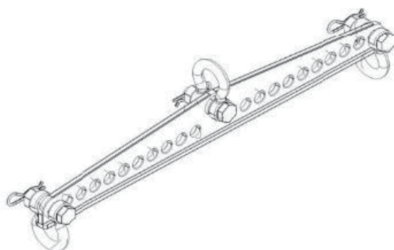
(図 15 : BAR-N-APS / N-APS 用水平アレイクラスターフレーム)
