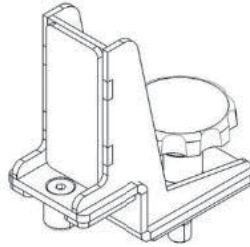
( 図 17 : GAH-N-APS / グラウンドスタッキングした N-SUB 上に N-APS の水平アレイを載せるときに使用するアダプター )
