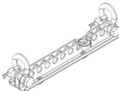
(図 13 : FRH-N-APS / N-APS 用水平アレイフレーム)
