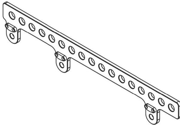
(図 16 EXBAR-AR : FR-AR/ FRT-AR 用エクステンションバー)
