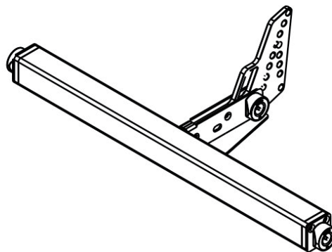
(図 18 CGA : CiRAY グランドスタックアダプター。 SC2-F/ SCV-F の上に最大 8 台まで CiRAY をスタックできる。)
