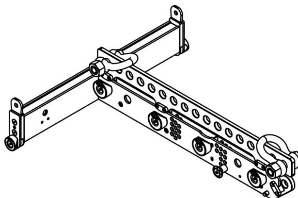
(図 15 FRT-AR-Set : AiRAY/ ViRAY/ CiRAY をフライングするためのフレーム)
