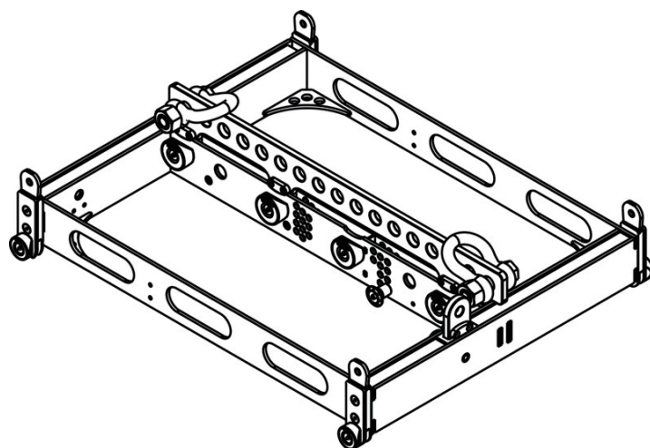
(図 14 FR-AR-Set : AiRAY/ ViRAY/ CiRAY/ SC2-F/ SCV-F をさまざまな組み合わせでフライングまたはグランドスタックするためのフレーム)
