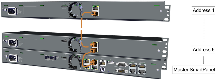
図 25 : ESP SmartPanel のデジチェーン接続
