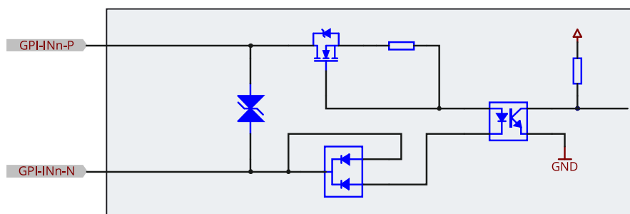
図 107 : GPI IN コネクタの回路図
