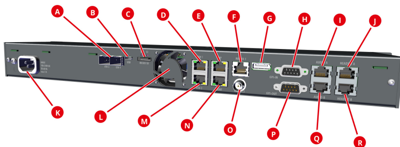
図 8 : RSP-1216HL 背面
