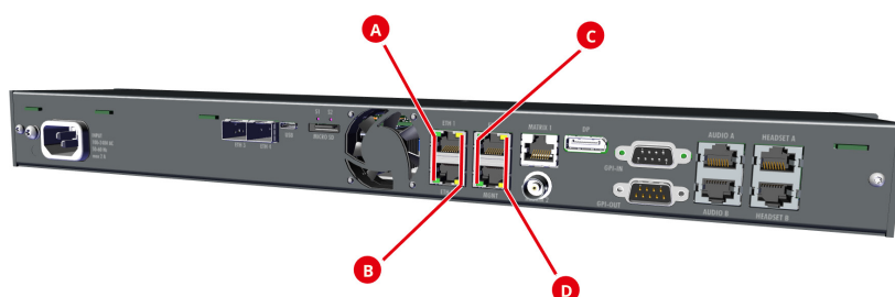
図 10 : RSP-1216HL 背面のステータス LED の位置
