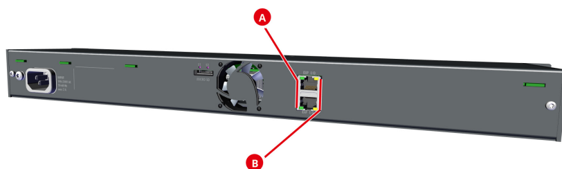
図 23 : ESP-1216HL 背面のステータス LED の位置
