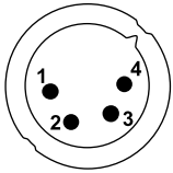
図 113: ヘッドセット・コネクタ (オス XLR-4) のピン割り当て
