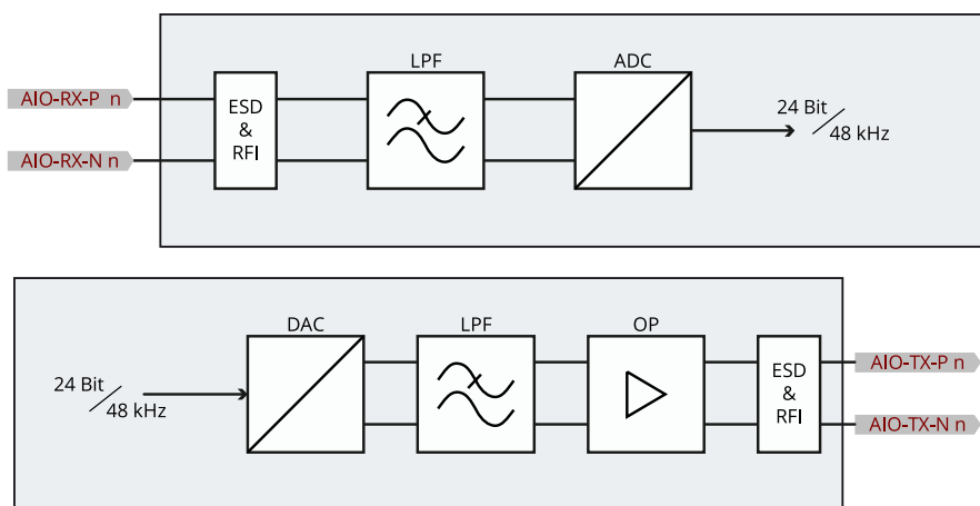
図 111 : 音声コネクタのブロック・ダイアグラム
