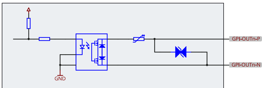
図 109 : GPI OUT コネクタの回路図
