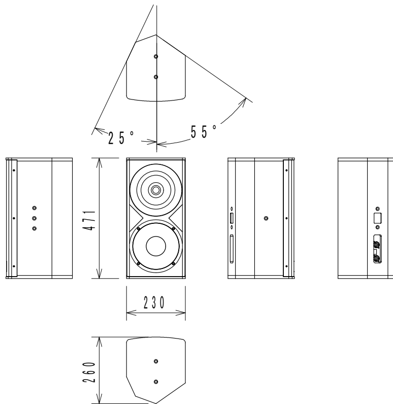
寸法図はG308-R (右側仕様)
