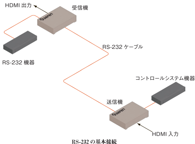
RS-232 の基本接続
