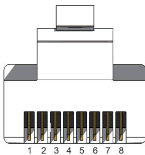
RJ-45 コネクターの前面
