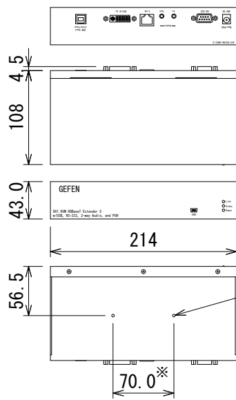
EXT-DVIKA-HBT2-S(送信機)
