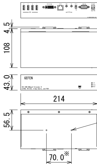
EXT-DVIKA-HBT2-R(受信機)
