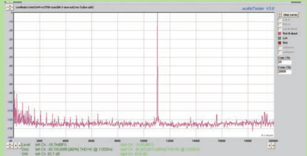
左の図と同じ構成で、MC-3 + USB を DAT レコーダと DAC 間の信号経路内に入れて測定。
