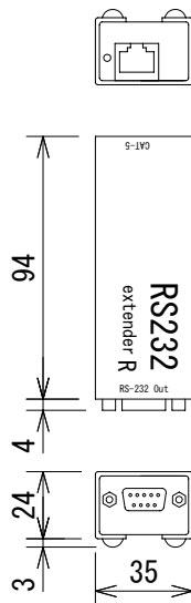
EXT-RS232 R(レシーバー)
