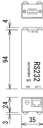
EXT-RS232 S(センダー)
