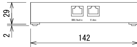
DVI AUDIO(レシーバー)
